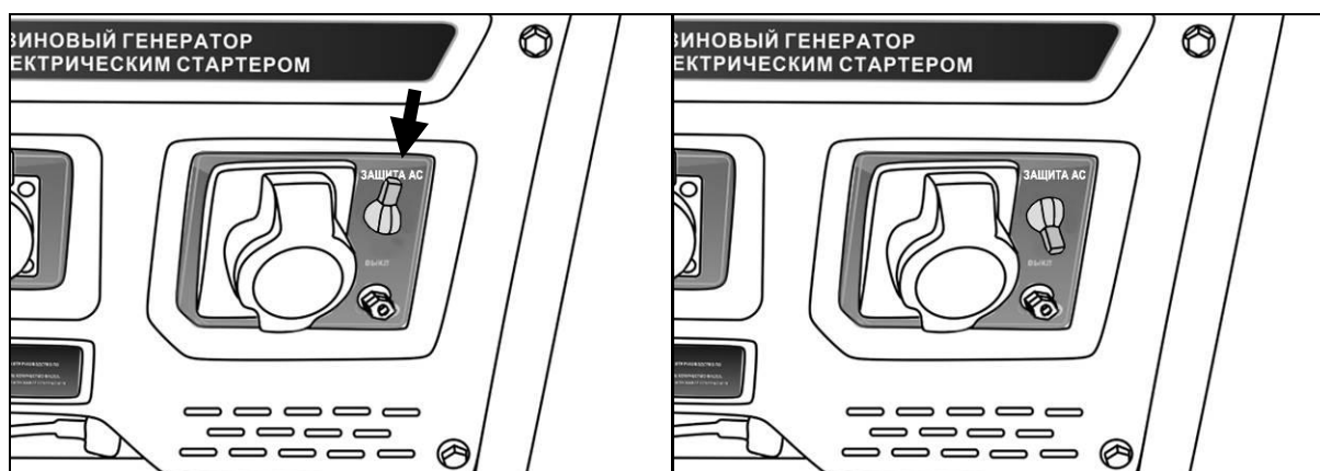
Рис. 12. Автоматический выключатель
